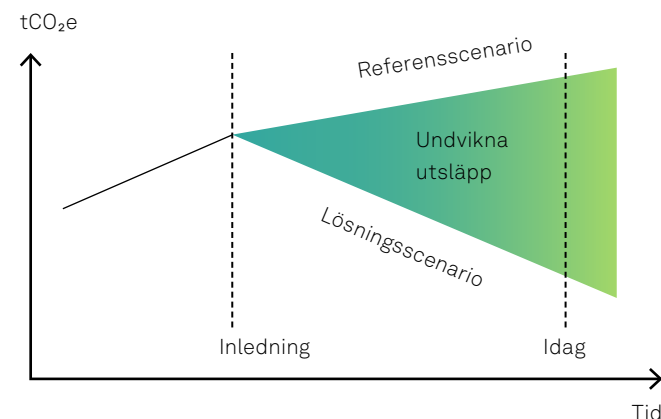
Figur 1 - Undvikna utsläpp
